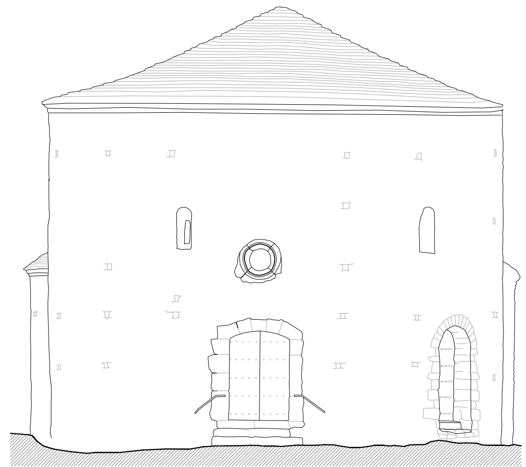
Alçat Nord-oest e 1/100
