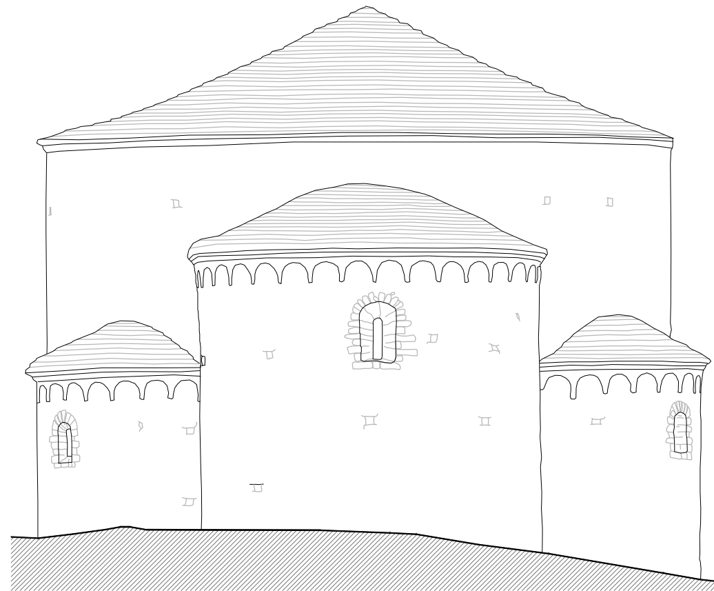
Alçat Nord-oest e 1/100
