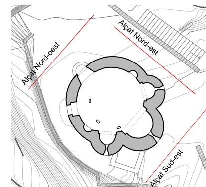
Planta església e 1/500
