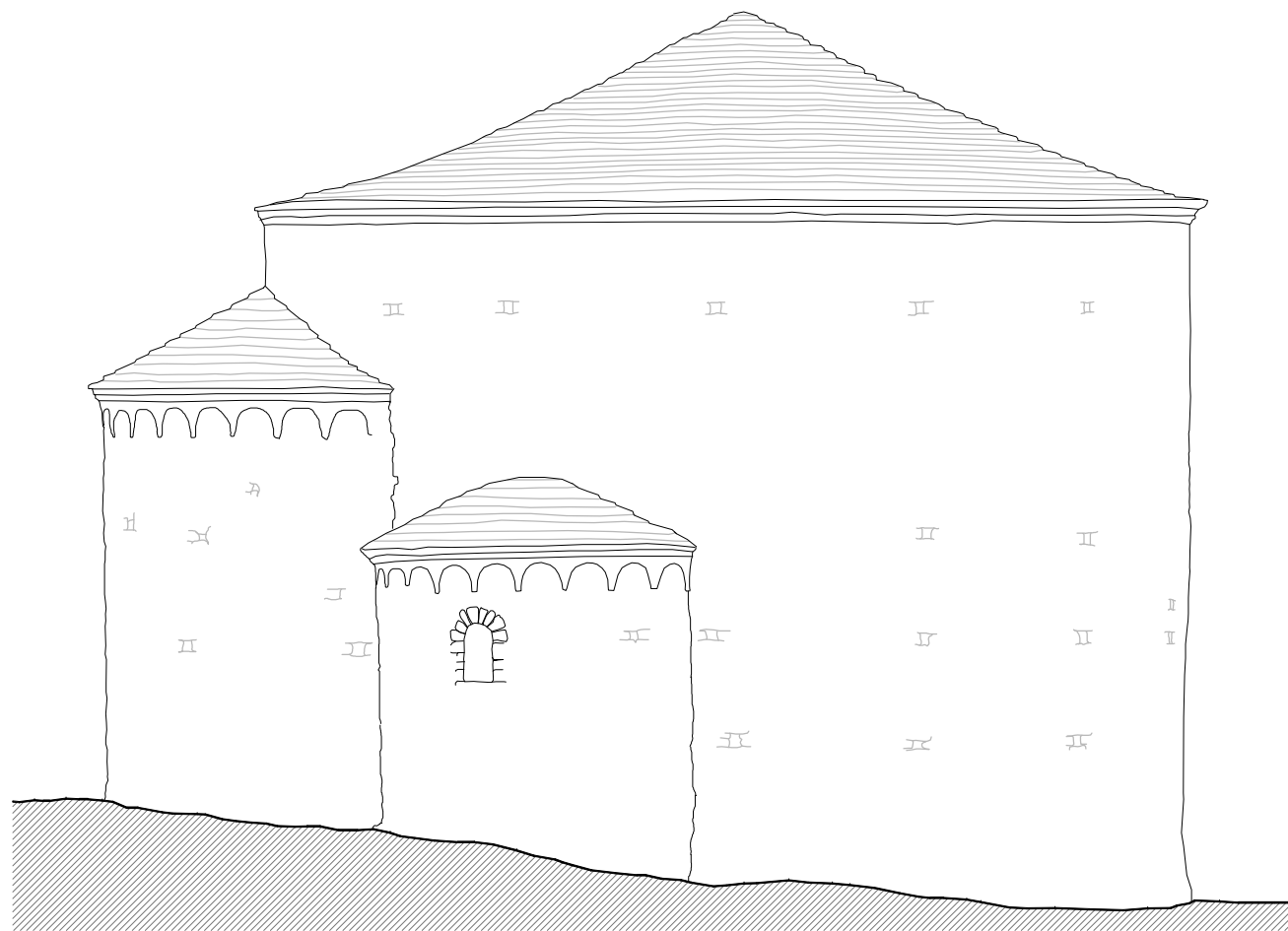
Alçat Nord-est e 1/100
